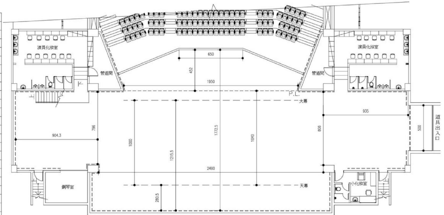
岡山演藝廳舞臺平面圖
